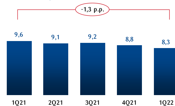
Wskaźnik dźwigni [%]
