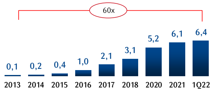
IKO [mln]
